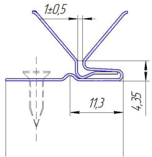
Состыковка профилей (2,5:1)
