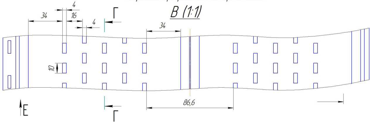
Вариант профиля №3 (с просечкой)
